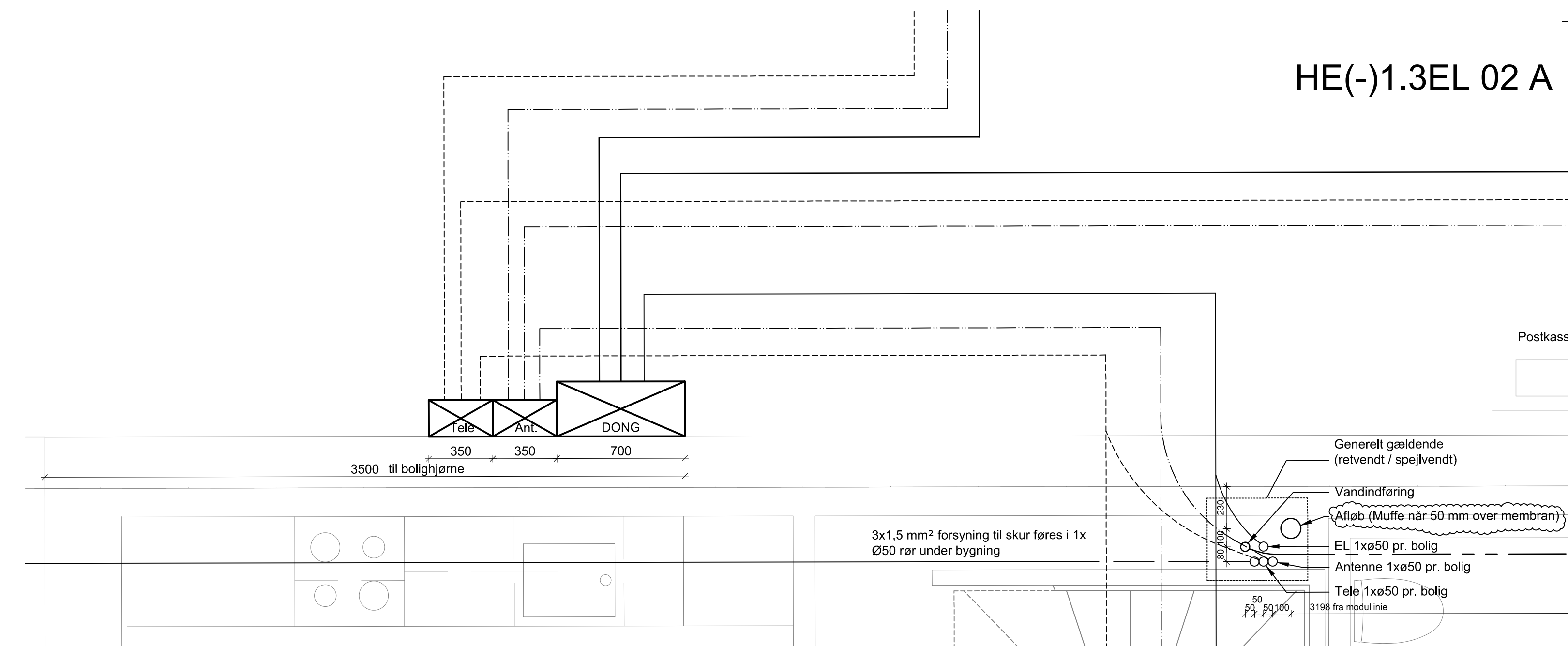
Deludsnit, 1:20
